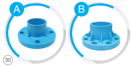
ប៊្រែដ - ក្រាស់ SOCKET WITH PVC FLANGE-WS B
